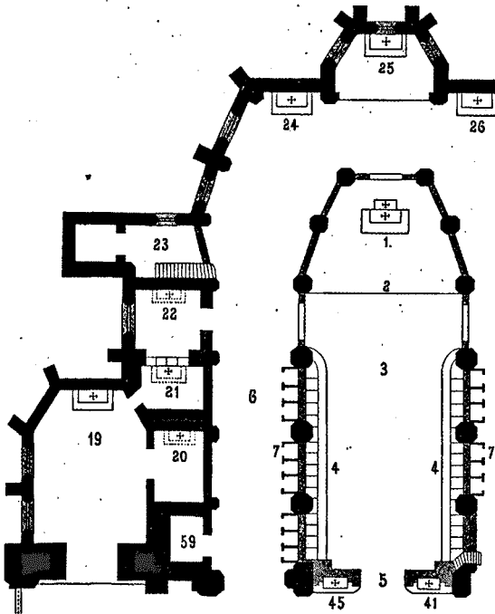
De noordelijke omgang van het koor van de Brugge O.L.Vrouwekerk in 1866: 59: opslagplaats, 19: de H. Kruiskapel, 20: H. Drieuldigheidskapel (Breydelkapel), (21)-22: St.-Margaretakapel (Bladelin of de Baenstkapel), 23: Gruuthuusekapel [18] .
